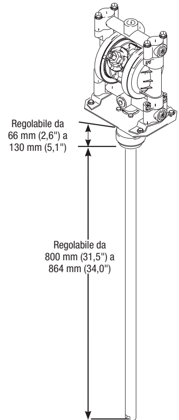
L'altezza totale dipende dalla pompa. Vedere pagina 12 o 15 per le dimensioni delle pompe.
