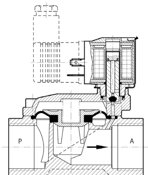
Sezione GEMÜ 8258
