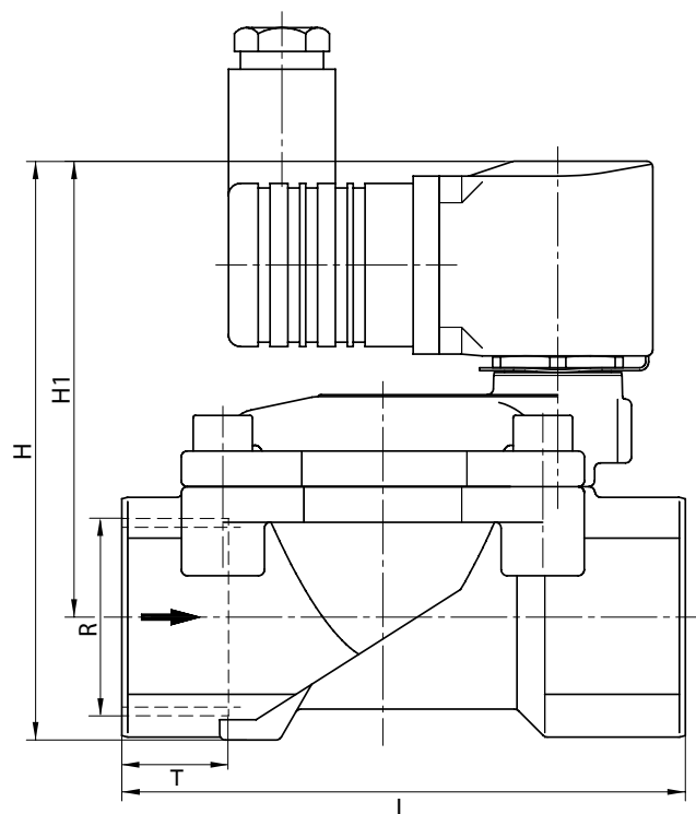
Dimensioni del corpo GEMÜ 8258 [mm]
